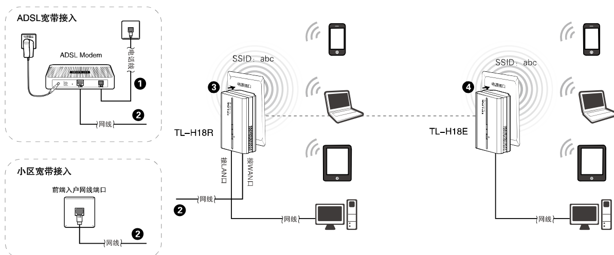
图 4-1 TL-H18R/TL-H18E 硬件安装示意图
